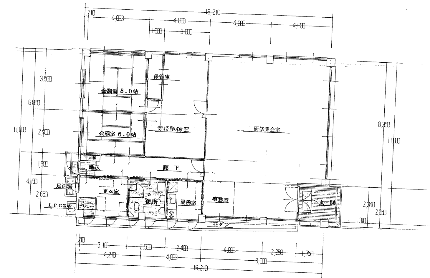
平面図
